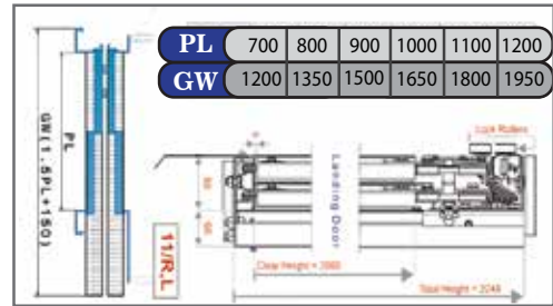
Çift teleskopik kapı
